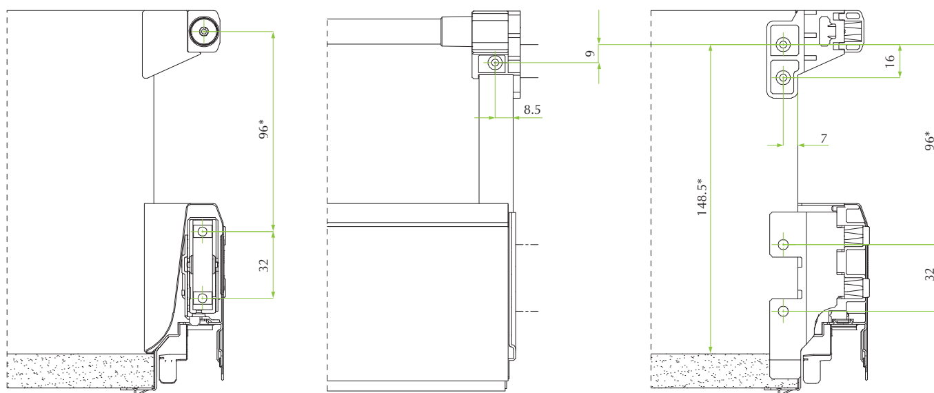
ВИД СПЕРЕДИ
