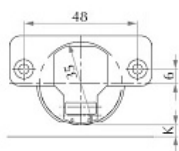
Схема сверления под чашку петли
