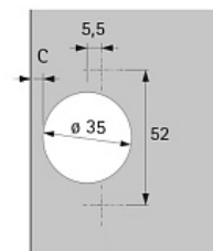
Карта сверления чашки петли
