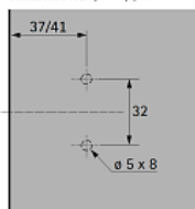
Присадка монтажной планки на фасадах
