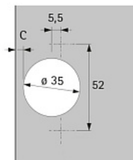
Карта сверления чашки петли
