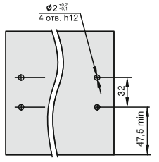
Размеры для крепления фиксаторов фасада на внутренней поверхности фасада
